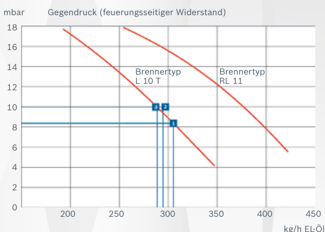
Grafik: Brenner-Kennfeld mit Maximalleistungskurven
