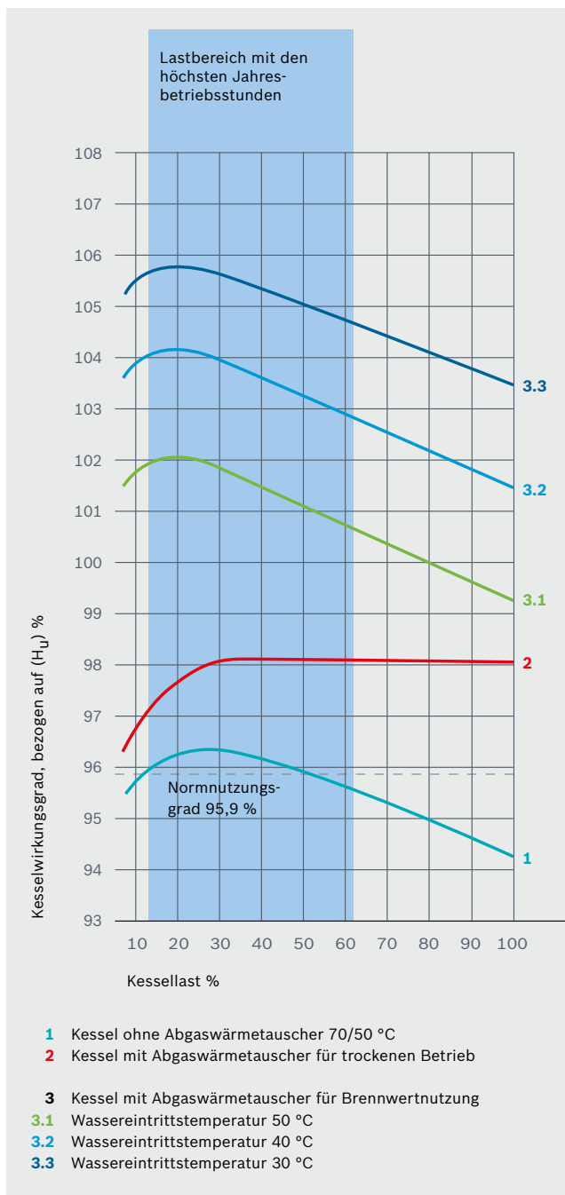
Grafik 2: Wirkungsgradkurven für UNIMAT Heißwasserkessel bei Kessel-Vorlauf/Rücklauf 70/50 °C
