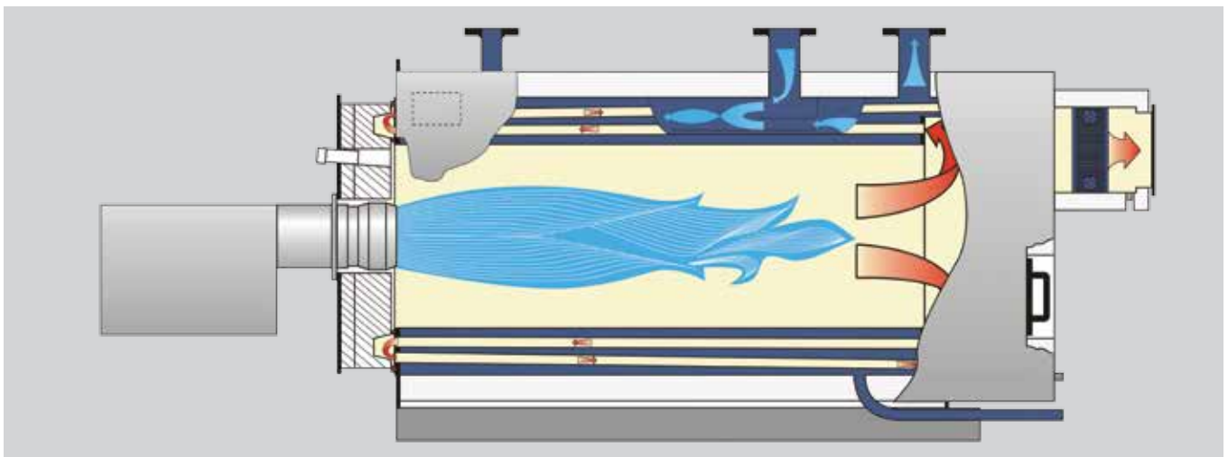
Abbildung 3: Einflamrohr-Rauchrohr-Heißwasserkessel im Dreizugprinzip mit Abgaswärmetauscher
