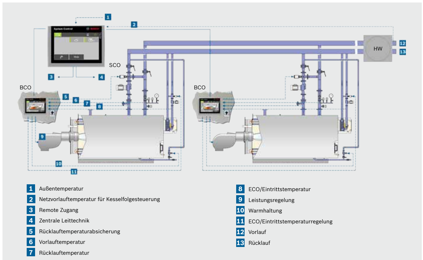
Abbildung 4: Witterungsgeführte Heißwasserkesselanlage mit hydraulischer Weiche
