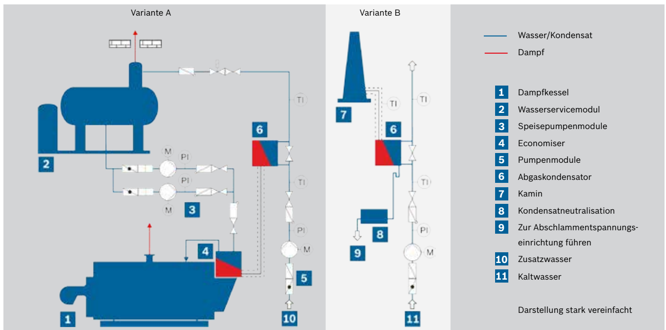
Abbildung 2: Dampferzeuger mit Zweistufenbetrieb – Economiser/Abgaskondensator; Brennstoffeinsparung bis zu 15 %
