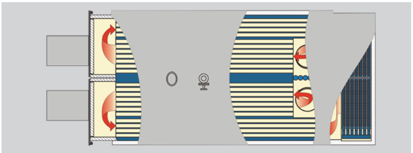
Abbildung 1: Zweiflammrohr-Rauchrohr-Dreizugkessel mit getrennten Rauchgaswegen für Brennereinzelnbetrieb und integriertem Economiser zur Speisewasseraufheizung
