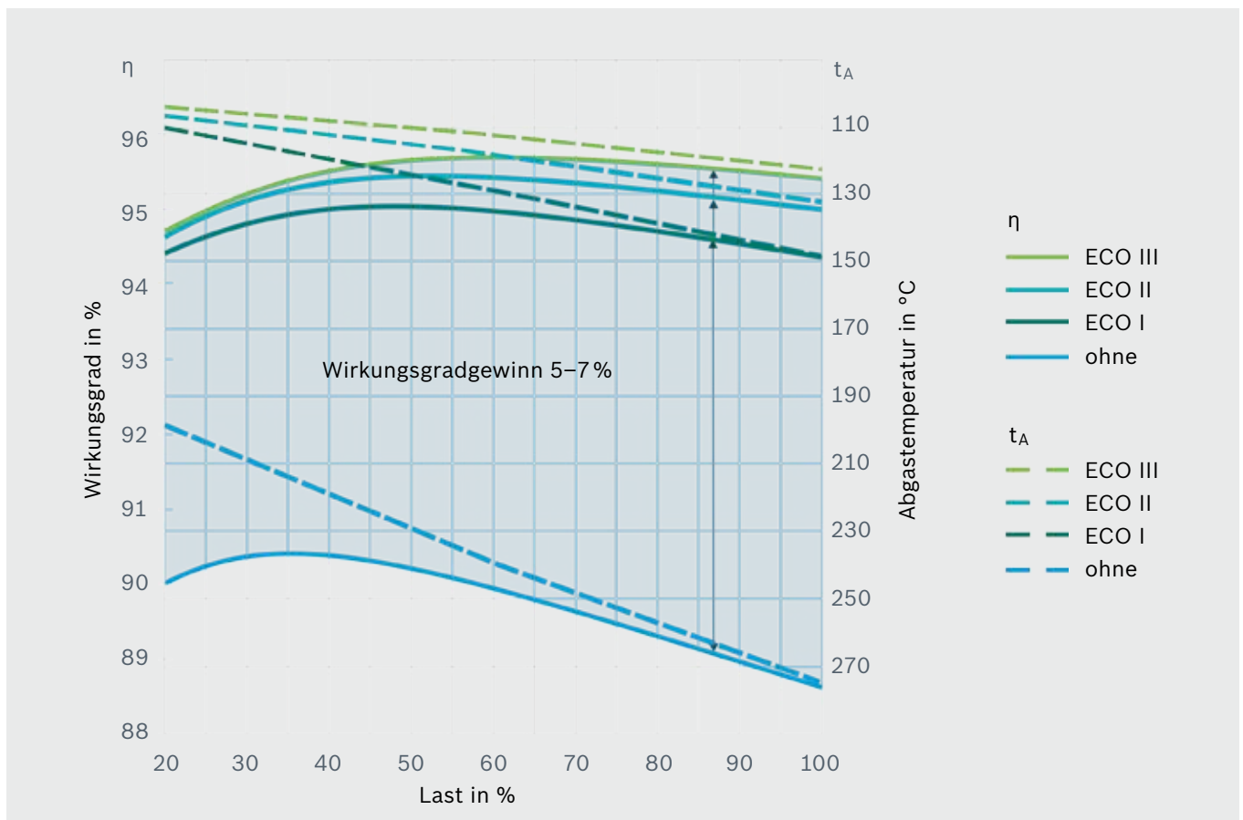
Grafik 1: Erzielbare Leistungsoptimierung durch Abgaswärmetauscher für „trockenen“ Betrieb
