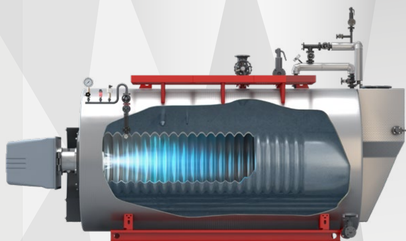
Bild 6: Schnitt durch einen modernen Dreizug-Dampfkessel mit eingebauten Elektrodensystem im Schutzrohr
