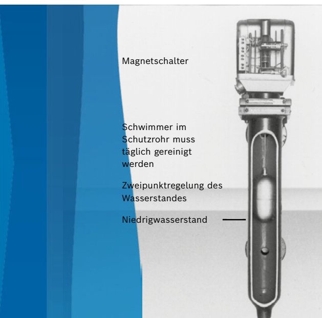
Bild 1: Schwimmer-Wasserstandsbegrenzer – das Prüfen der Sicherheitsschaltung und das tägliche Durchblas-Reinigen sind vorgeschrieben
