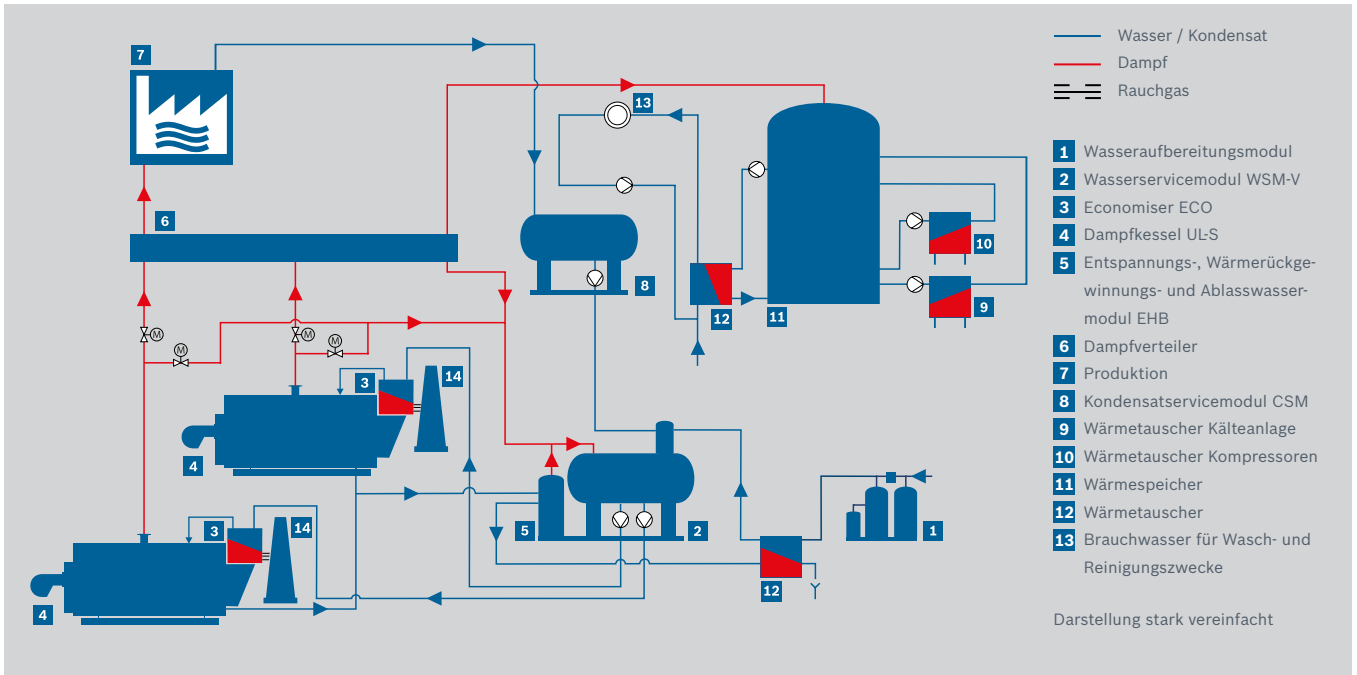
Systembild Dampfkessel mit entsprechender Anlagentechnik zur Wärmerückgewinnung, Wasseraufbereitung und Kondensatrückführung sowie Abwärmenutzung der Kompressoren und Kühllhäuser.
