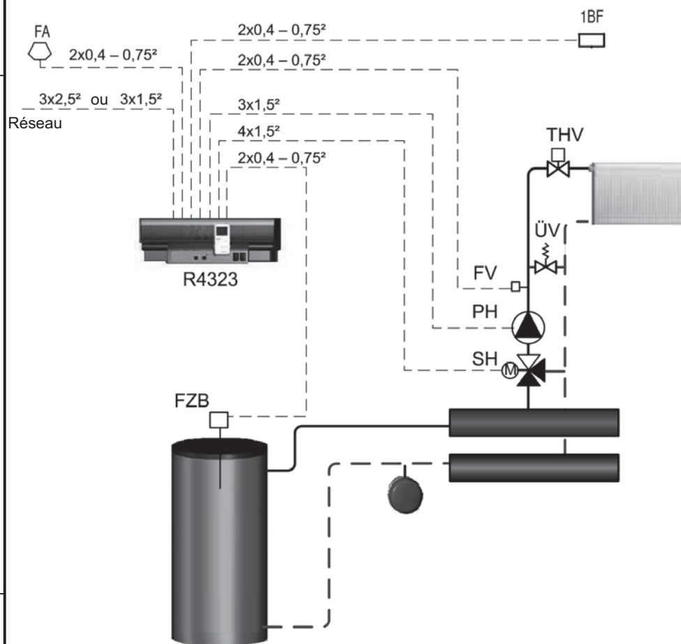
Installation de chauffage en autarcie
