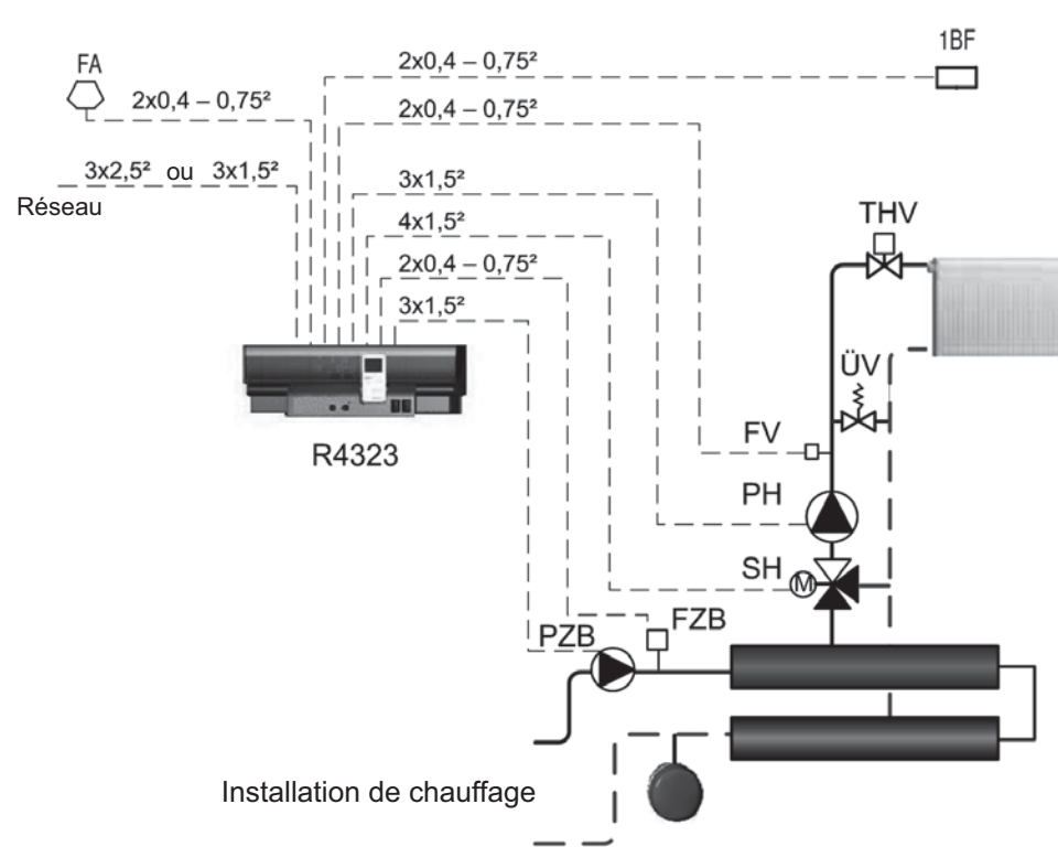
Exemple d'installation 2
