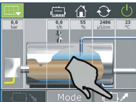
Figure 3 : Commande du BCO (Boiler Control) – le démarrage automatique de la chaudière est assuré par une pression sur l'icône de l'écran tactile « Démarrer » ou un signal externe.
