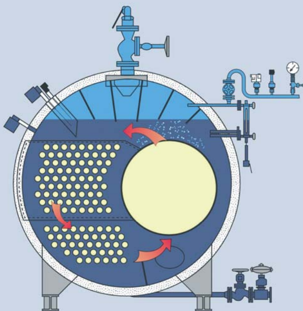
Figure 1 : Représentation schématique de la circulation naturelle mise en œuvre dans la chaudière, dans la mesure où une évacuation de la vapeur est permise durant la procédure de démarrage.
