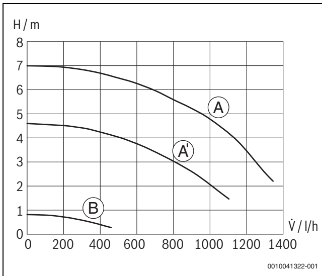
Bild 3 Pumpenkennfeld
